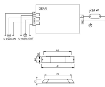
Technische Daten Philips HID-PV m 35 /I CDM 220-240V 50/60Hz für 35W
